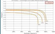
不同環境溫度下LYP類電池的放電特性曲線 LFP battery's discharge curve under different temperatures
